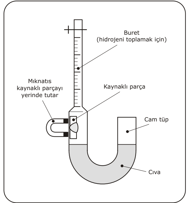
Şekil-5 Yayınabilir Hidrojen İçin Ölçme Düzenneği
